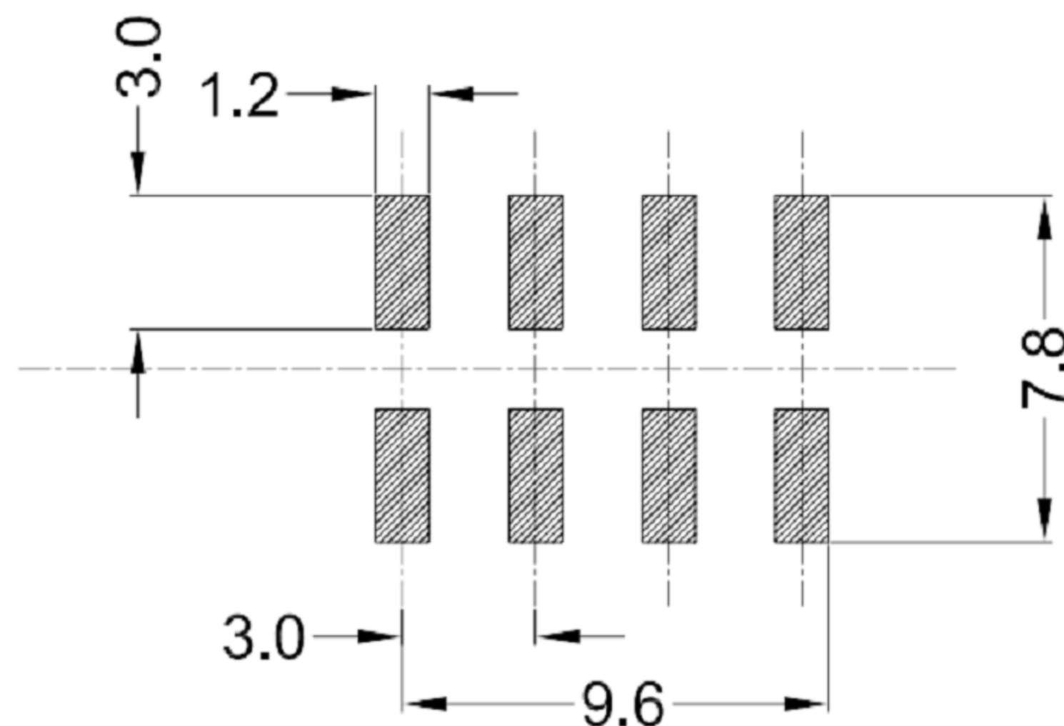
P.C.B LAYOUT
